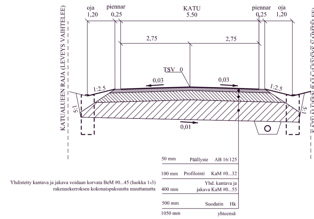
Rakenteellinen tyyppipoikkileikkaus 1:100
