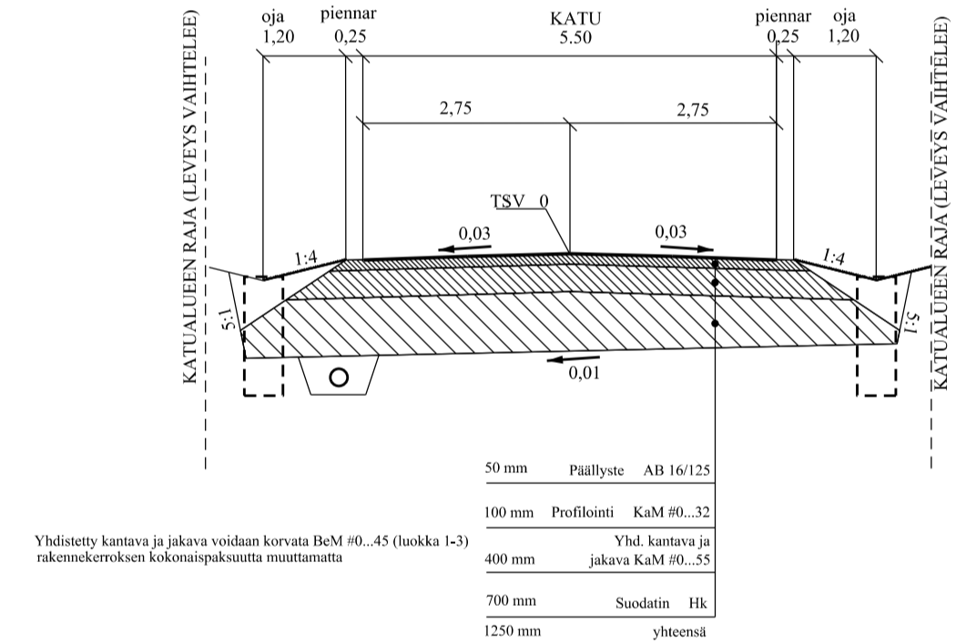
Rakenteellinen tyypipoikkileikkaus 1:100
