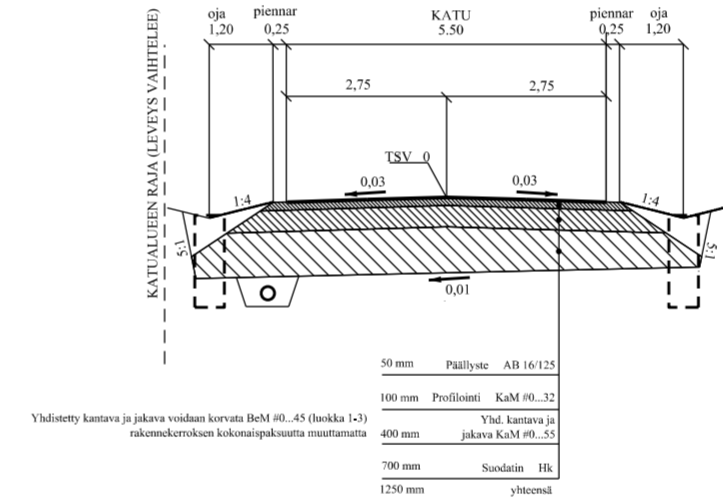
Rakenteellinen tyypipoikkileikkaus 1:100
