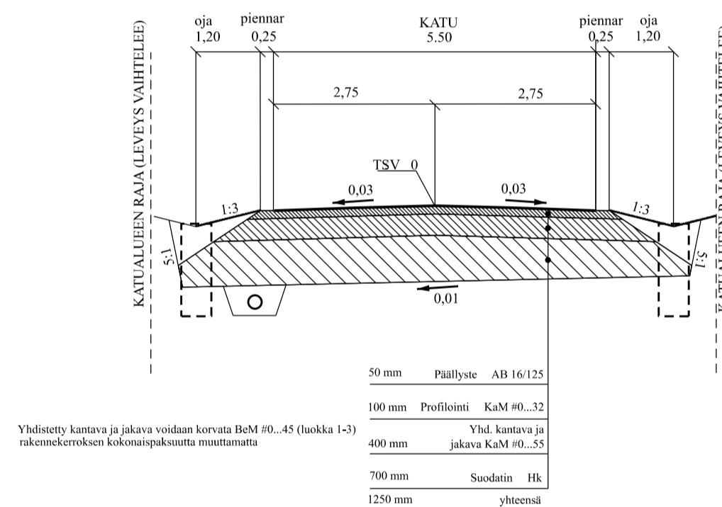
Rakenteellinen tyyppipoikkileikkaus 1:100
