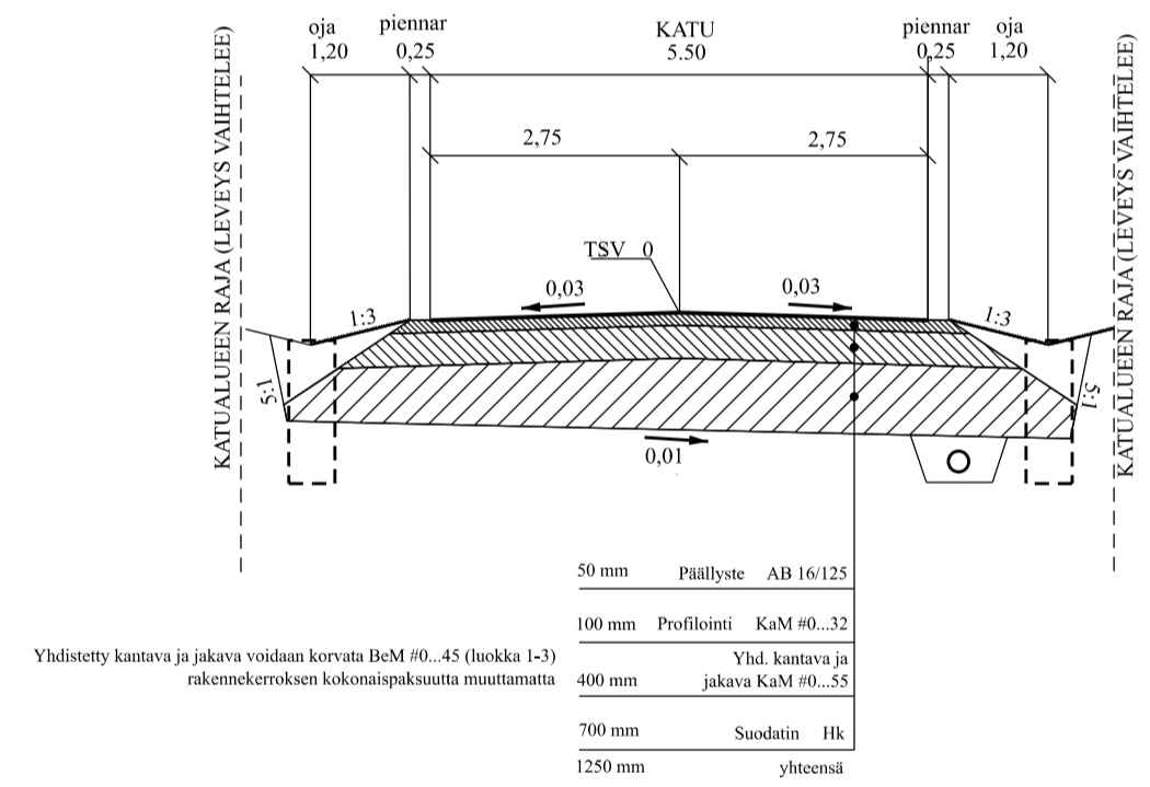
Rakenteellinen tyyppiokileikkaus 1:100
