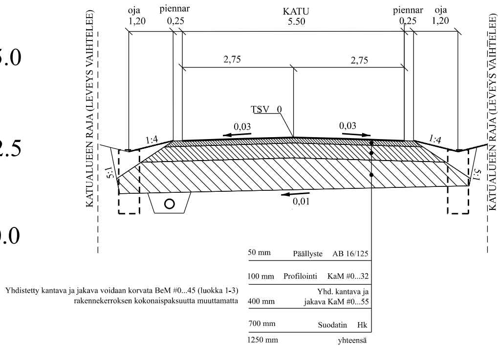
Rakenteellinen tyypipoikkileikkaus 1:100
